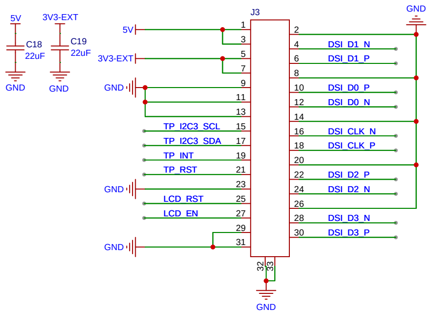
MIPI_DSI
